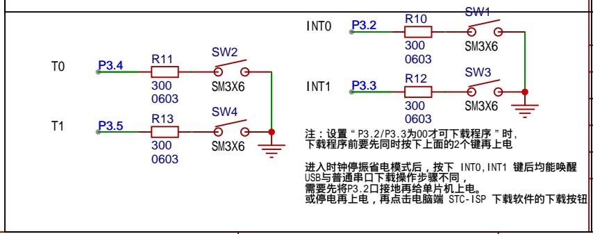
AI8051U主控电路
