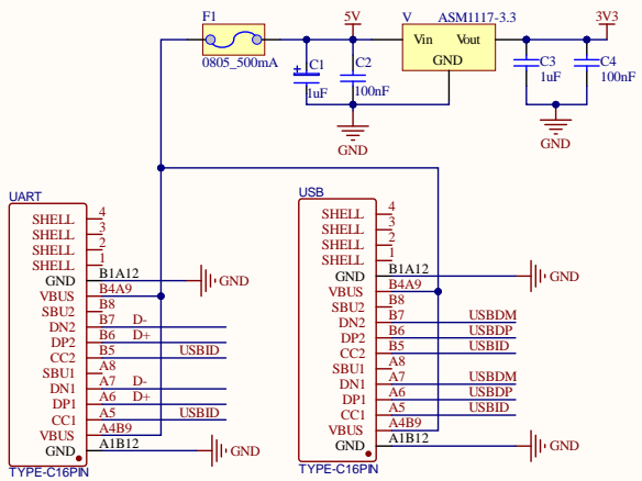
供电/下载/仿真调试电路接口
