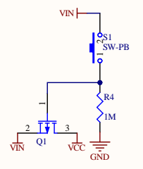
冷启动/复位电路
