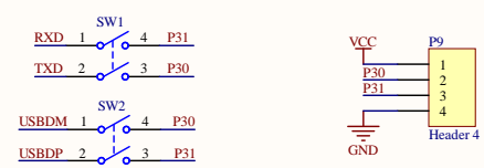
USB通信/串口通信→切换
