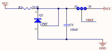
基准电源电路
