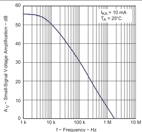
图 6-10. 小信号电压放大与频率之间的关系
