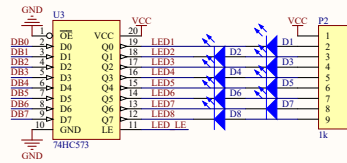
流水灯
