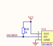
DS18B20
