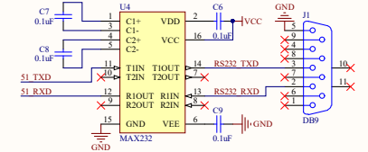
MAX232
