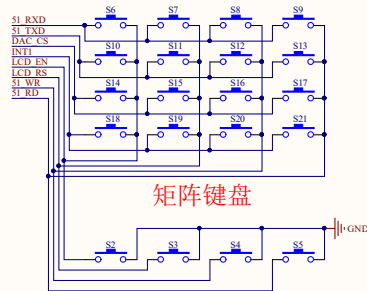
独立按键
