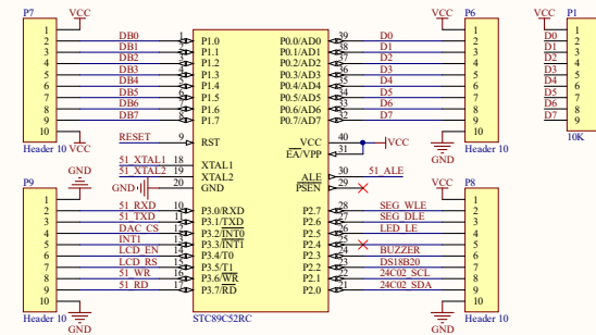
MCU 最小系统
