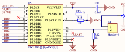
ADC
