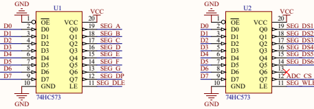
数码管
