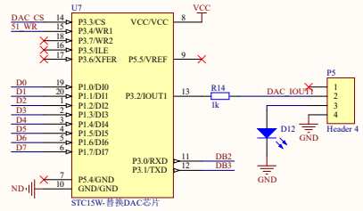
DAC
