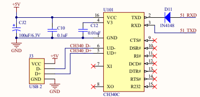
CH340C 下载
