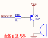
蜂鸣器
